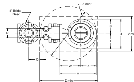
DIMENSIONES CODO DE DESCARGA VISTA INFERIOR
